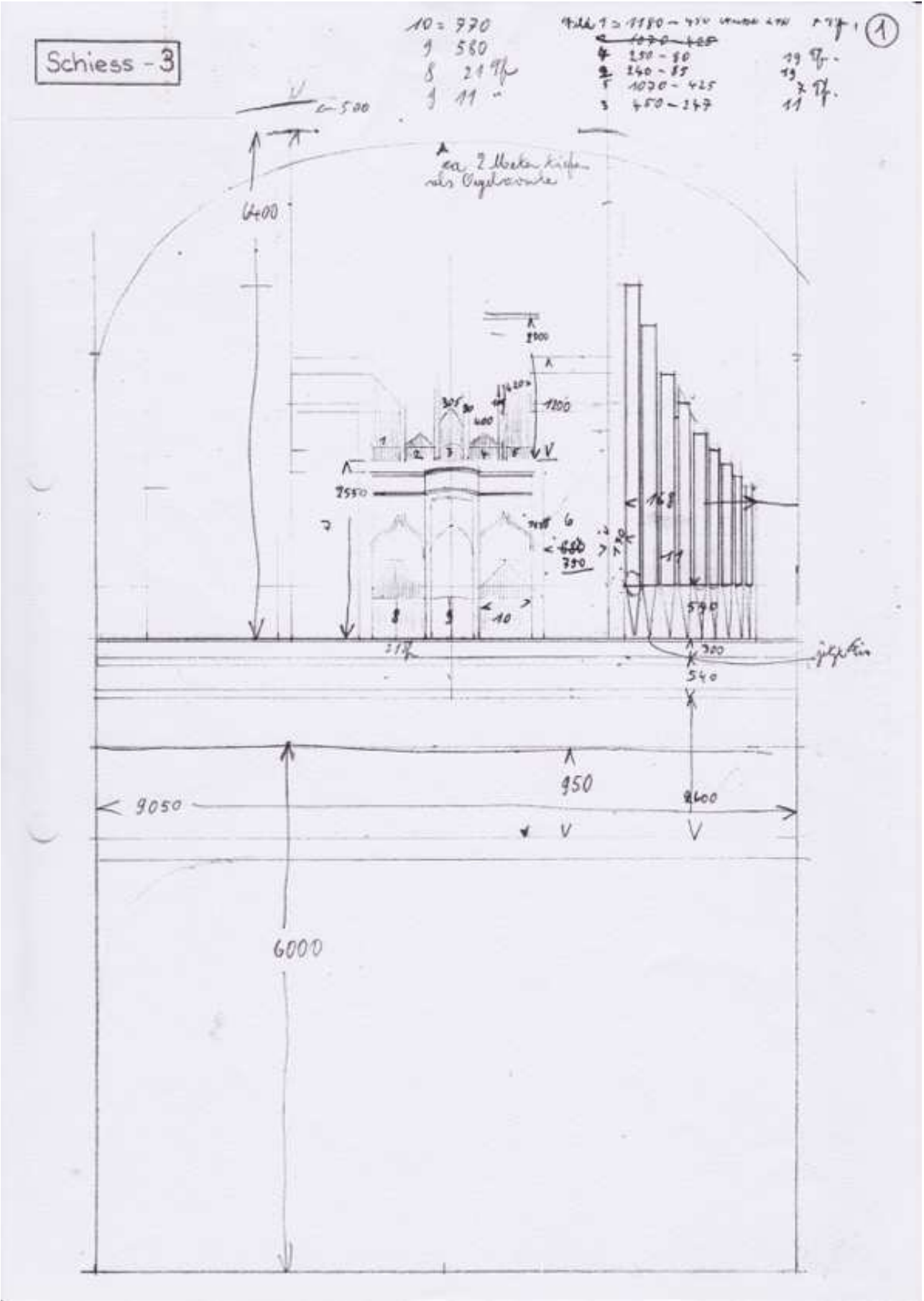
Abb. 9: Schiess-3,1: Goll-Orgel, Bestandesaufnahme von 1938, Blatt 1.
